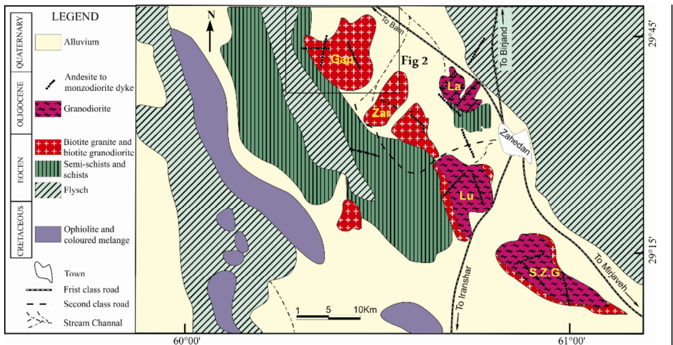
شکل ۱ پراکندگی و ترکیب توده‌های گرانیتوئیدی پیرامون زاهدان که در فلیش‌های ائوسن نفوذ کرده‌اند. این نقشه از رضائی کهنائی و همکاران [۶] برگرفته شده است. (Gap: گپدان، Zar: زرگلی، La: لخشک، Lu: لوچان و S.Z.G: گرانیتوئیدهای جنوب زاهدان).
