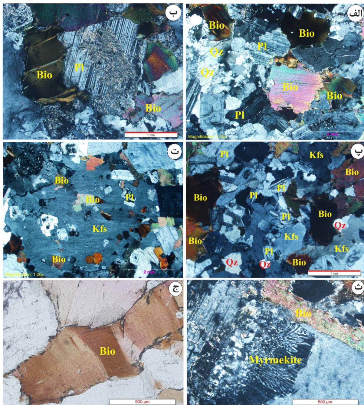
شکل ۳ الف) تصویر میکروسکوپی از بیوتیت گرانیت‌های توده گیدان. ب) تجزیه پلاژیوکلازهای موجود در بیوتیت گرانیت‌ها به سریسیت. پ) تصویر میکروسکوپی از گرانودیوریت‌های همان توده و کانی‌های موجود در آن‌ها. ت) میانبرهای کوچک پلاژیوکلاز و بیوتیت داخل پتاسیم فلدسپار. ث) هم‌رشدی کانی‌های پلاژیوکلاز و کوارتز و ایجاد بافت میرمکیتی. ج) خمیدگی بلورهای بیوتیت در اثر تحمل دگربرختی حالت جامد. این پدیده بیشتر در سنگ‌های حاشیه توده گیدان مشاهده می‌شود.
