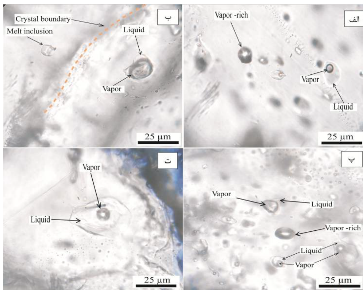
شکل ۷ تصاویر میکروسکوپی انواع مختلف میانبارهای سیال اولیه در کانسار طلای زرشوران: الف) میانبارهای سیال دوفازی مایع (L+V) و تک فاز غنی از بخار (V)، ب) میانبارهای سیال دو فازی غنی از بخار (V+L) با فراوانی بسیار کم، که میانبار مذاب این تصویر نتیجه به تله افتادن مذاب موجود در سیال گرمایی کانه‌زاست، پ) میانبارهای سیال تک‌فازی مایع (L) و بخار (V) همراه با میانبارهای سیال دوفازی غنی از مایع (L+V)، و ت) میانبار سیال اولیه دو فازی غنی از مایع و بی‌شکل.
