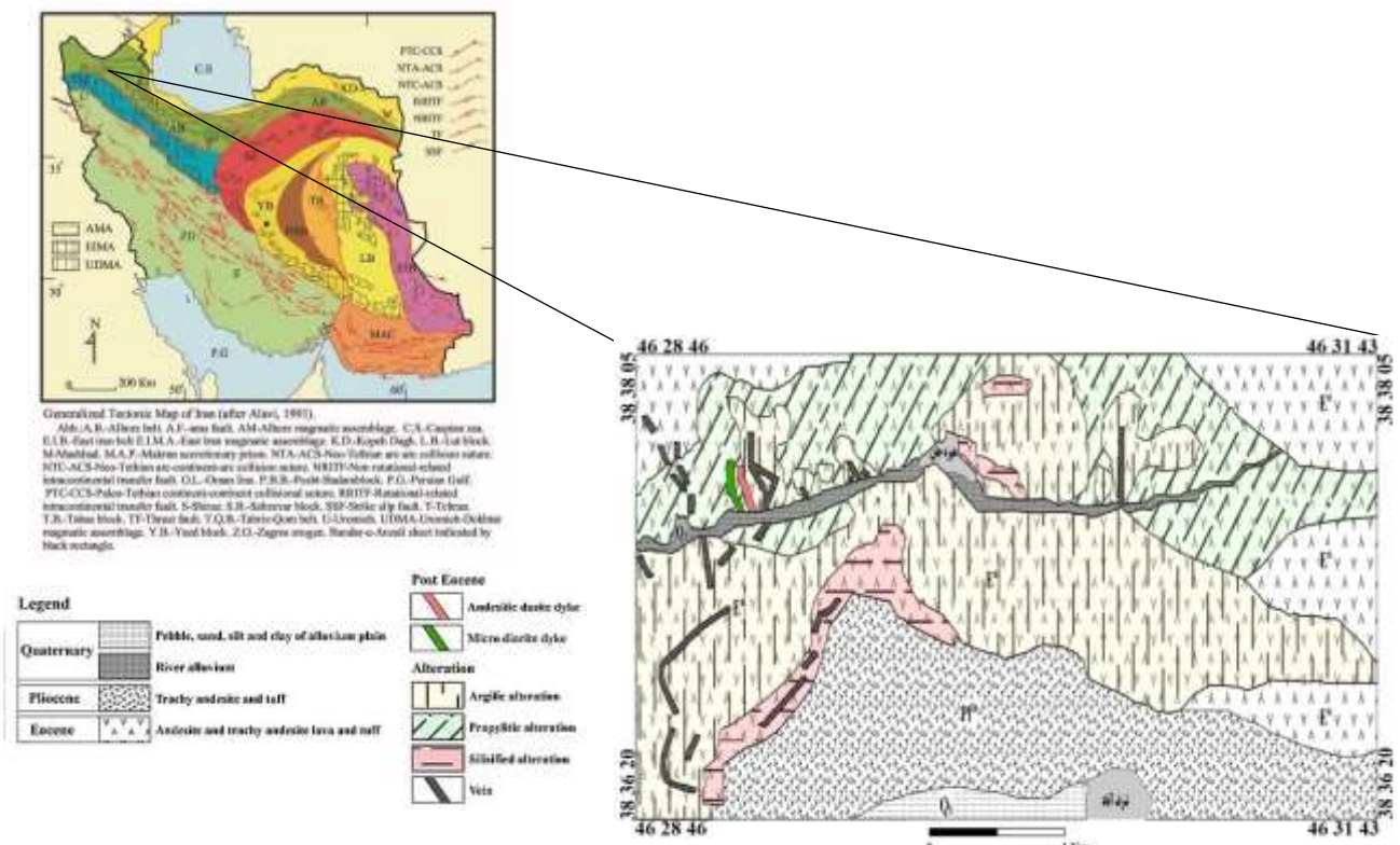
شکل ۱ نقشه زمین‌شناسی - دگرسانی برگرفته از مراجع ۱۸۱-۱۱۵ با اندکی تغییرات که منطقه مورد بررسی بر اساس تقسیم بندی مرجع [۱] در پهنه البرز- آذربایجان (AB) و زیر پهنه مجموعه ماگمایی البرز (AMA) قرار دارد. رگه‌ها صرفاً جهت نمایش در نقشه آورده شده است.
