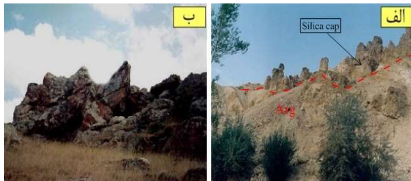
شکل ۸ الف- کلاهک سیلیسی در بخش بالایی پهنه آرژیلی که به دلیل افزایش سیلیس دارای ریختار خشن است. دید به سمت شمال غرب ب- رگه‌های ژاسپیروئیدی که شامل سیلیس دانه‌ریز با آغشتگی اکسید آهن است. دید به سمت جنوب.
