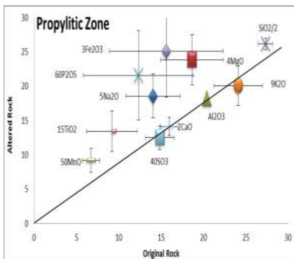
شکل ۹ نمایش تغییرات الف) عناصر اصلی و ب) فرعی بصورت ایزوکن در پهنه پروپلیتی.
