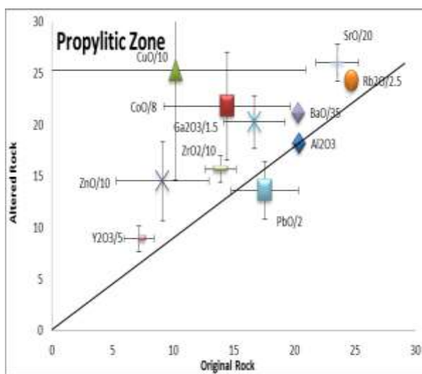
شکل ۹ نمایش تغییرات الف) عناصر اصلی و ب) فرعی بصورت ایزوکن در پهنه پروپلیتی.
