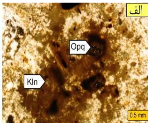
شکل ۱۲ تبدیل فلدسپار به کانی های رسی کائولینیته و مونت موریلونیتی و ایجاد دگرسانی آرژیلی. (نور XPL): Kln : کانی های رسی کائولینیته و مونت موریلونیتی، Opq : کانی های کدر. علائم کانی ها بر اساس مرجع [۱۹].
