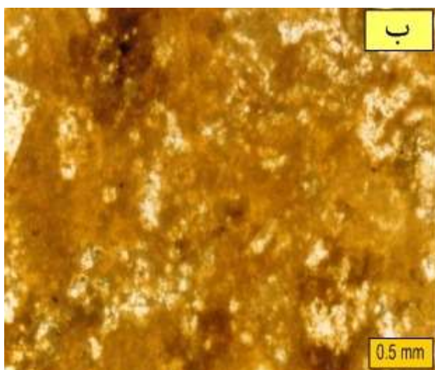
شکل ۱۲ تبدیل فلدسپار به کانی های رسی کائولینیته و مونت موریلونیتی و ایجاد دگرسانی آرژیلی. (نور XPL): Kln : کانی های رسی کائولینیته و مونت موریلونیتی، Opq : کانی های کدر. علائم کانی ها بر اساس مرجع [۱۹].
