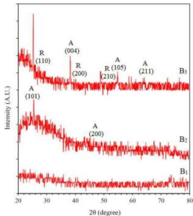
شکل ۷ طیف پراش پرتو X (XRD) از نمونه‌های B_1 ، B_2 و B_3
