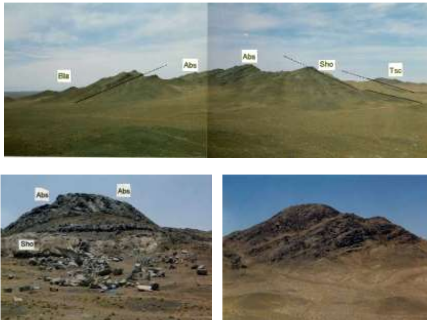
شکل ۴ تصاویر صحرایی مجموعه شوشونیتی قلعه خرگوشی. افساروکیت‌ها، شوشونیت‌ها، باناکیت یا لاتیت‌ها، و توسکانیت‌ها به ترتیب با علائم Abs، Sho، Bla، و Tsc نشان داده شده‌اند.
