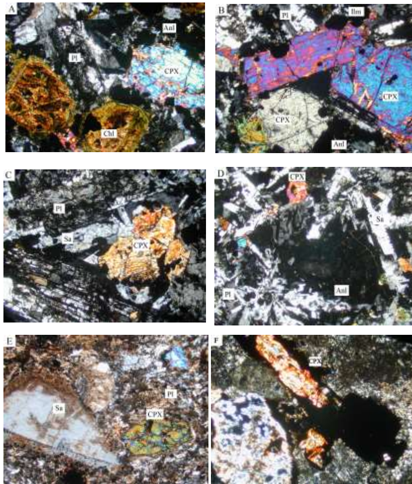
شکل ۵ تصاویر سنگ‌شناسی سنگ‌های سری شوشونیتی منطقه قلعه خرگوشی.
