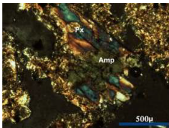
شکل ۱۲ هوادیدگی پیروکسن (Px) به آمفیبول (Amp) در افق Bt2 بدون ۲- سمت راست XPL و چپ PPL.
