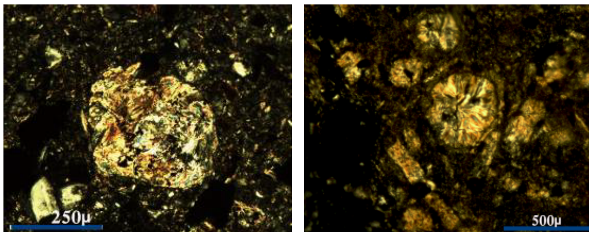
شکل ۱۰ هوادیدگی اولیوین به کلریت در افق Bt1 (سمت راست) و افق A (سمت چپ) بدون ۲- XPL.
