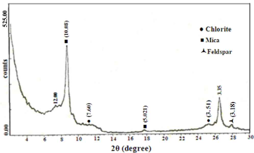
شکل ۱۱ پراش نگاشت پرتو ایکس رس افق A (تیمار K-110) بدون ۲.
