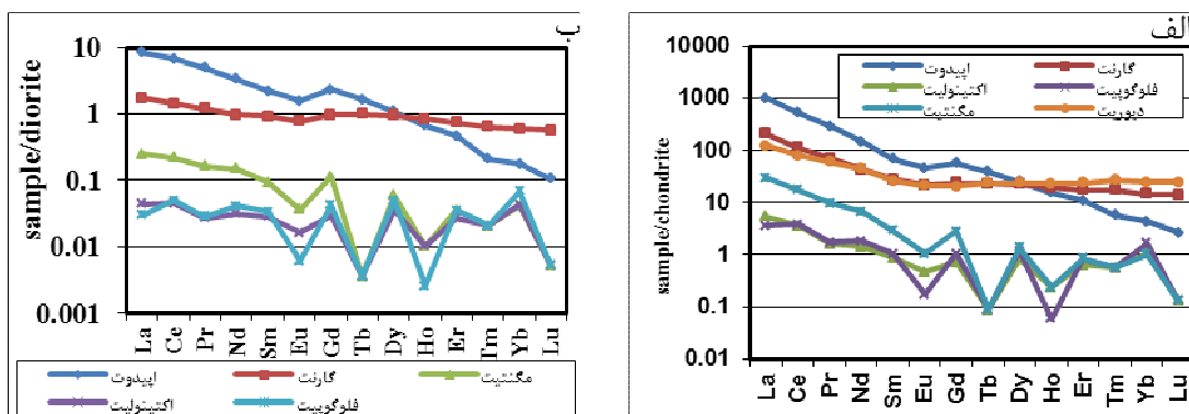
شکل ۱۰ فراوانی عناصر خاکی نادر در کانی‌ها الف) بهنجار شده با کندریت‌ها [۶] ب) بهنجار شده با دیوریت میزان.
