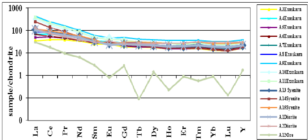
شکل ۴ فراوانی عناصر خاکی نادر در نمونه‌های اگزواسکارنی، سینیتی، دیوریتی و منطقه‌ی معدنی بهنجار شده با کندریت‌ها [۶].
