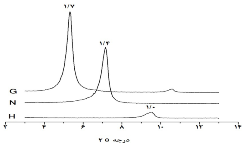
شکل ۱ پراش نگاشت پرتو ایکس وابسته به کانی بنتونیت مورد استفاده در بررسی (الف) نمونه‌ی پودری، (ب) نمونه‌ی تیمار شده با اتیلن گلیکول + منیزیم اشباع و گرمادهی (C: کلسیت، Mt: مونتموریلونیت، Q: کوارتز؛ G: اشباع با منیزیم + اتیلن گلیکول، N: اشباع با منیزیم، H: اشباع با پتاسیم + گرمادهی با دمای ۵۳۰ درجه سانتیگراد، اعداد قله‌ها بر حسب نانومتر هستند).
