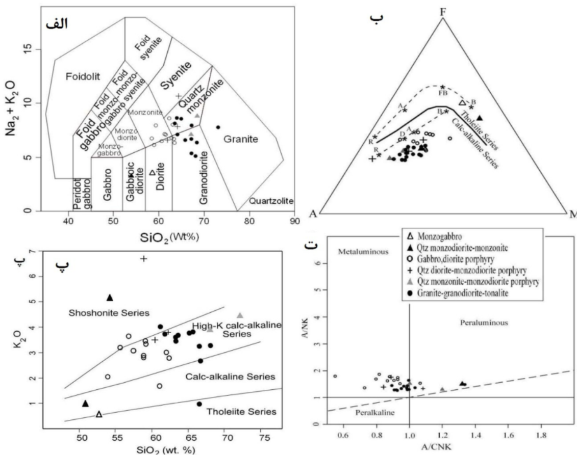
شکل ۵ موقعیت توده‌های نفوذی و نیمه عمیق کاشمر در: الف) نمودار Na_2O+K_2O در برابر SiO_2 [۲۳]، ب) نمودار AFM [۲۴]، پ) نمودار K_2O در برابر SiO_2 [۲۵]، ت) نمودار تعیین اندازه آلومینیوم (A/NK-A/CNK) [۲۶].
