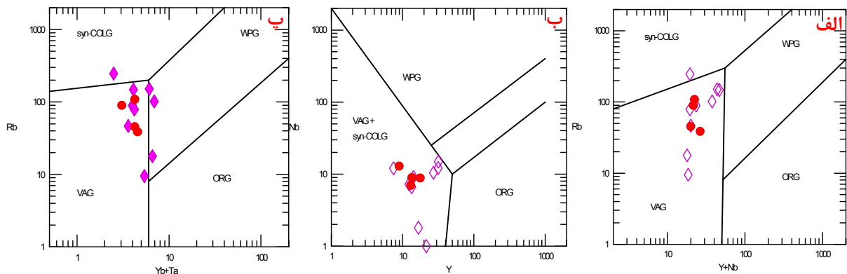
شکل ۱۲ الف، ب و پ) نمودارهای تعیین موقعیت زمین‌ساختی با استفاده از نمودار Rb در مقابل Nb در مقابل Y، Rb در مقابل Yb+Ta در مقابل Yb+Ta [۴۲] بنابر این نمودارها، نمونه‌های مورد بررسی بیشتر در قوس‌های آتشفشانی قرار می‌گیرند (VAG). (ORG = مناطق پشته‌ای اقیانوسی = VAG = مناطق کمان آتشفشانی WPG = مناطق داخل صفحه‌ای COLG = محیط‌های تصادمی) (نمادهای لوزی سنگ‌های درونی و نمادهای دایره سنگ‌های بیرونی).
