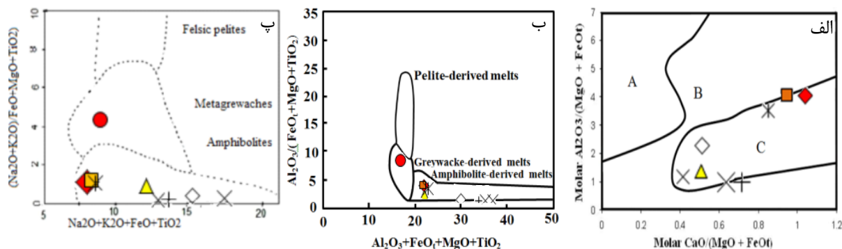
شکل ۱۴ الف) نمودار تعیین خاستگاه سنگ‌های مورد بررسی [۴۵] که بر این نمودار، نمونه‌های مورد بررسی در گستره‌ی شبه‌بازالت‌ها و شبه-تونالیت‌ها واقع شده‌اند (A: گدازه با خاستگاه متاپلیتی، B: گدازه با خاستگاه متاگربوکی، C: گدازه با خاستگاه متابازالتی و متانوالیتی). ب و پ) نمودار تعیین نوع سنگ خاستگاه بر پایه‌ی اکسیدهای Al_2O_3/(FeO+MgO+TiO_2) در مقابل Al_2O_3+FeO+MgO+TiO_2 و (Na_2O+K_2O)/(FeO+MgO+TiO_2) در مقابل Na_2O+K_2O+TiO_2 [۴۵] که مذاب‌هایی با منشأ آمفیبولیتی را نشان می‌دهند (نمادها مشابه با شکل ۶-الف).
