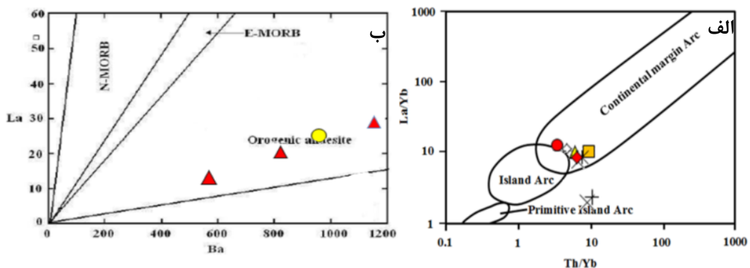
شکل ۱۳ الف) نمودار La/Yb در مقابل Th/Yb [۴۳] برای تعیین محیط زمین‌ساختی توده‌های گرانیتوئیدی مورد بررسی (نشانه‌ها مشابه با شکل ۶-ب) تعیین محیط زمین‌ساختی سنگ‌های بیرونی منطقه مورد بررسی [۴۴] بنابر این نمودار، سنگ‌های منطقه‌ی مورد بررسی در گستره‌ی آندزیت‌های ناشی از کوهزایی قرار می‌گیرند (نمادها مشابه با شکل ۶-ب).
