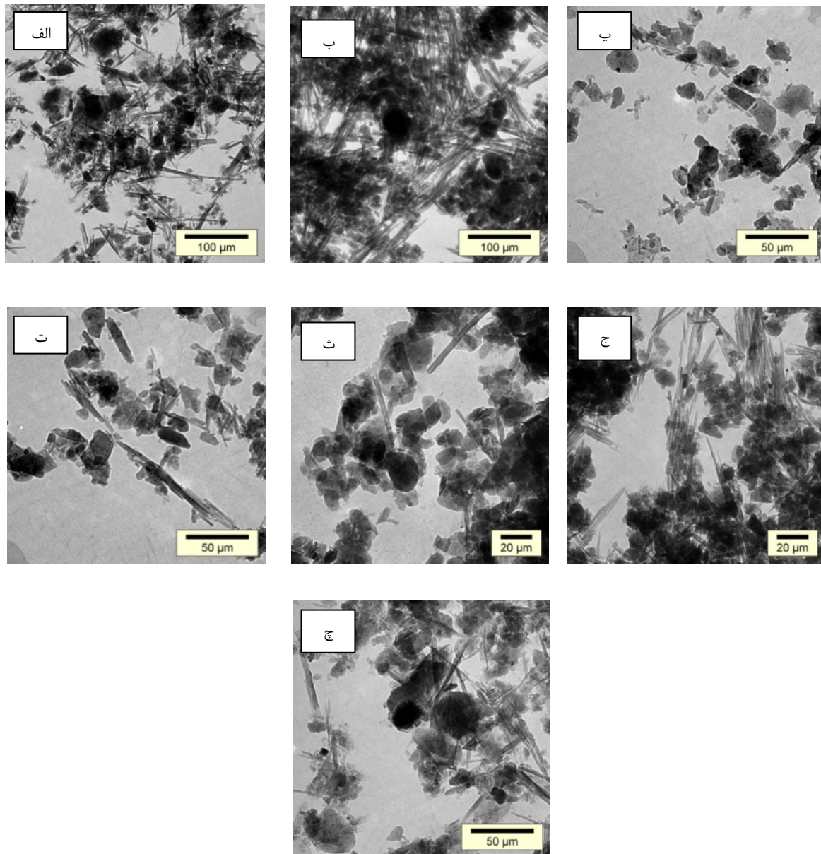
شکل ۴ ریزنگاشت میکروسکوپ الکترونی عبوری افق‌های By2 (الف) و Btmyz (ب) خاکرخ ۱، Az (پ) و Btmyz (ت) خاکرخ ۲، Az (ث)، By2 (ج) و C (چ) خاکرخ ۳ نشان دهنده بلورهای دسته جارویی و منفرد پالیگورسکیت
