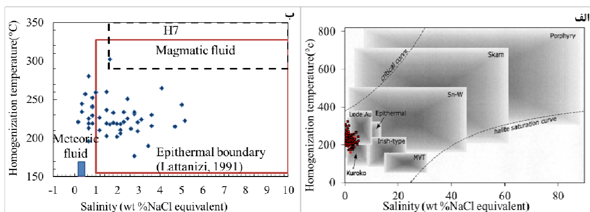
شکل ۷ الف) موقعیت نمونه های مزرعه شادی در نمودار شوری نسبت به دمای همگن شدگی [۲۲] ب) نمودار شوری نسبت به دمای همگن شدگی در گمانه H۷ بر اساس نتایج مراجع [۲۳-۲۵].
