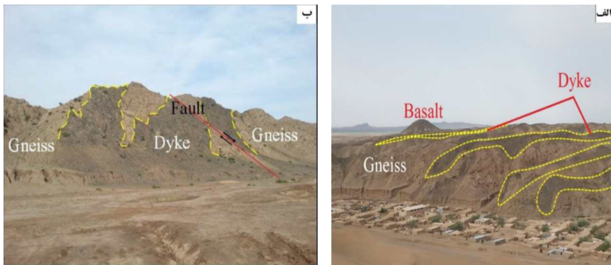
شکل ۳ الف) نمایی از دسته دایک‌های دیابازی قطع کننده واحد گنیسی در غربی روستای رضآباد (دید به سمت جنوب غربی). ب) نمایی از دایک‌های رضا آباد که توسط گسل راستگرد جابه‌جا شده است (دید به سمت شمال غربی).
