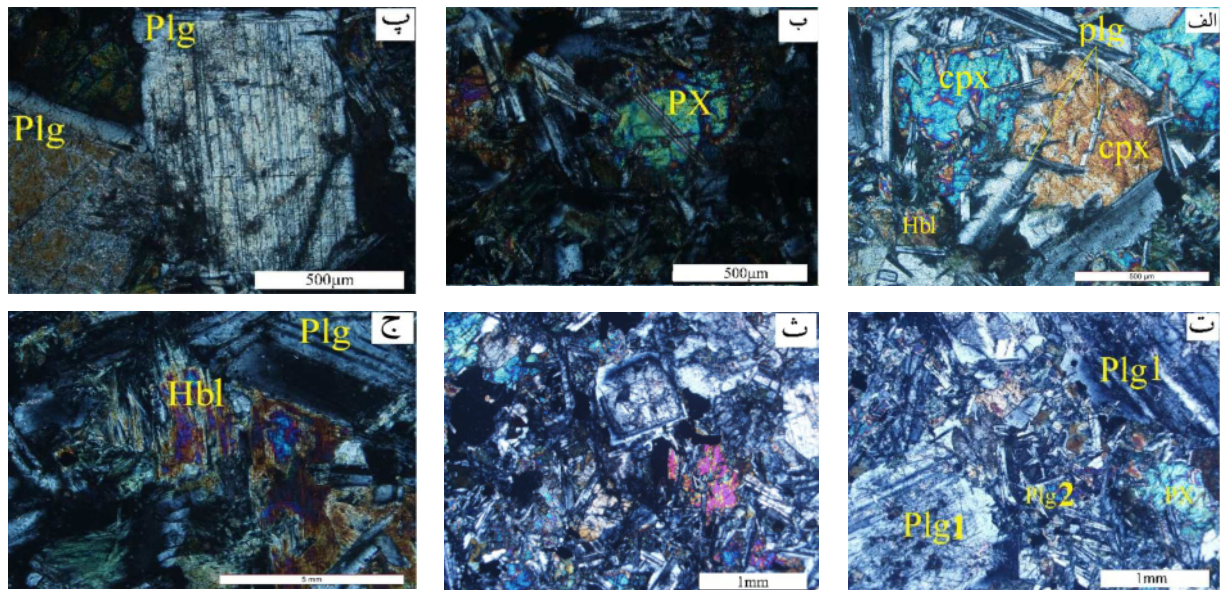
شکل ۴ الف) نمایش بافت افیتی و نیمه افیتی در دایک‌های دیابازی (ب) تصویری از بلور کلینوپیروکسن با ماکل اوزیتی (XPL)، (پ) ماکل پلی- سنتتیک در پلاژیوکلازها (XPL)، (ت) تصویری از وجود دو نسل پلاژیوکلاز در نمونه‌های دیابازی (XPL)، (ث) منطقه‌بندی در درشت بلور پلاژیوکلازهای نسل اول (XPL)، (ج) تصویری از کانی هورنبلند در دایک‌های دیابازی که در حال تبدیل شدن به کلریت است (XPL).
