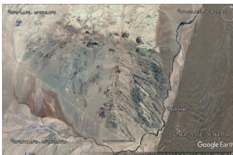
شکل ۲ تصویر هوایی گوگل از دسته دایک‌های دیابازی با روند تقریبی شمال غربی - جنوب شرقی.
