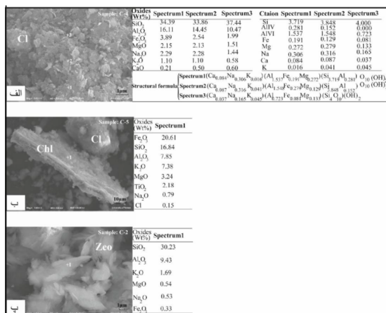
شکل ۵: آنالیزهای SEM-EDS از رس‌ها. (الف) ترکیب برخی از اکسیدهای اصلی در سه نقطه از اسمکتیت‌ها، (ب) ترکیب برخی از اکسیدهای اصلی در یک نقطه از کلریت‌ها و (ث) ترکیب برخی از اکسیدهای اصلی در یک نقطه از زئولیت‌های تشتاب.
