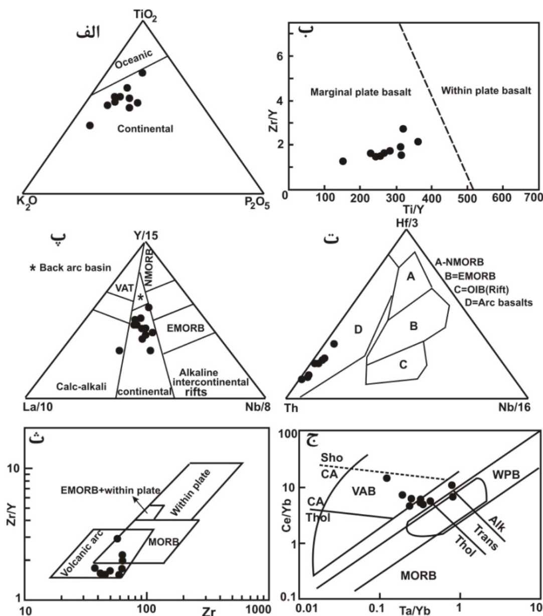
شکل ۹. بنابر نمودارهای جداکننده‌ی جایگاه زمین‌ساختی متداول و مرسوم، جایگاه متابازیت‌های مجموعه‌ی دگرگونی گشت، بازالت حاشیه فعال (قاره‌ای؟) بوده است. الف) با توجه به نمودار مثلی [۲۸]، جایگاه پروتولیت متابازیت‌های مجموعه دگرگونی گشت قاره‌ای است. ب) در نمودار دوتایی نسبت Ti/Y در برابر Zr/Y [۲۹]، تمام نمونه‌ها در گستره‌ی بازالت‌های حاشیه‌ی فعال قاره‌ای واقع شده‌اند. پ) بنابر نمودار مثلی- Y/15 Nb/8-La/10 [۳۰] متابازیت‌های مورد بررسی، ویژگی‌های ژئوشیمیایی بازالت قاره‌ای را نشان می‌دهند. ت) با توجه به نمودار مثلی [۳۱]، پروتولیت نمونه‌های مورد بررسی بازالت کمان آتشفشانی است. ث) در نمودار دوتایی جداکننده‌ی جایگاه‌های زمین‌ساختی کمان آتشفشانی، پشته‌ی میان اقیانوسی و داخل صفحه‌ای [۳۲]، جایگاه متابازیت‌های مجموعه‌ی دگرگونی گشت کمان آتشفشانی است. ج) در نمودار دوتایی نسبت Ta/Yb در برابر Ce/Yb [۳۳]، نمونه‌های مورد بررسی غالباً در گستره‌ی بازالت‌های کمان آتشفشانی یا مجاور آن واقع شده‌اند.
