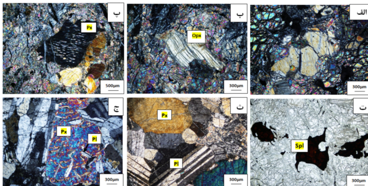
شکل ۳ الف: حضور بلورهای الیون و ارتوپروکسن. ب: خمیدگی رخ های ارتوپروکسن در پریدوتیت. پ: تیغه های عدم آمیزی کلینوپروکسن به موازات رخ های ارتوپروکسن در پریدوتیت. ت: کروم اسپینل در پریدوتیت. ث: ماکل کوتاه شونده در پلاژیوکلاز درون گابرو. ج: قرارگیری پلاژیوکلاز درون پیروکسن در گابرو. شکل های الف، ب، پ، ث، ج، در نور متقاطع (XPL) و شکل ت در نور موازی (PPL) گرفته شده اند. علائم اختصاری با اقتباس از [۲۸] عبارتند از: Pl = پلاژیوکلاز، Px = پیروکسن، Opx = ارتوپروکسن، Spl = اسپینل.
