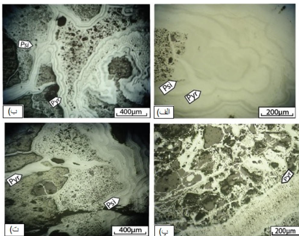
شکل ۵ الف، ب) بافت کلوتید در بخش مرکز شکل‌های کلو فورم پسیلوملان و اطراف آن پیرولوسیت تشکیل شده است (ppl)، پ، ت) بافت پرکننده فضای خالی که شکستگی‌ها به‌وسیله‌ی پیرولوسیت پر شده است (ppl).
