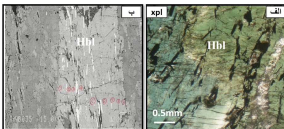
شکل ۸ (الف) تصویر میکروسکوپی هورنبلند (Hbl) سبز-آبی گلوگاه در نمونه‌ی B3، (ب) تصویر BSE هورنبلند آنالیز شده در نمونه‌ی B3 با مقیاس 100μm.
