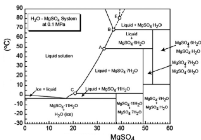
شکل ۸ نمودار سامانه \text{MgSO}_4 - \text{H}_2\text{O} در ۰/۱ Mpa برای نمایش محدوده پایداری کانی‌های سولفاتی منیزیم [۱۳].
