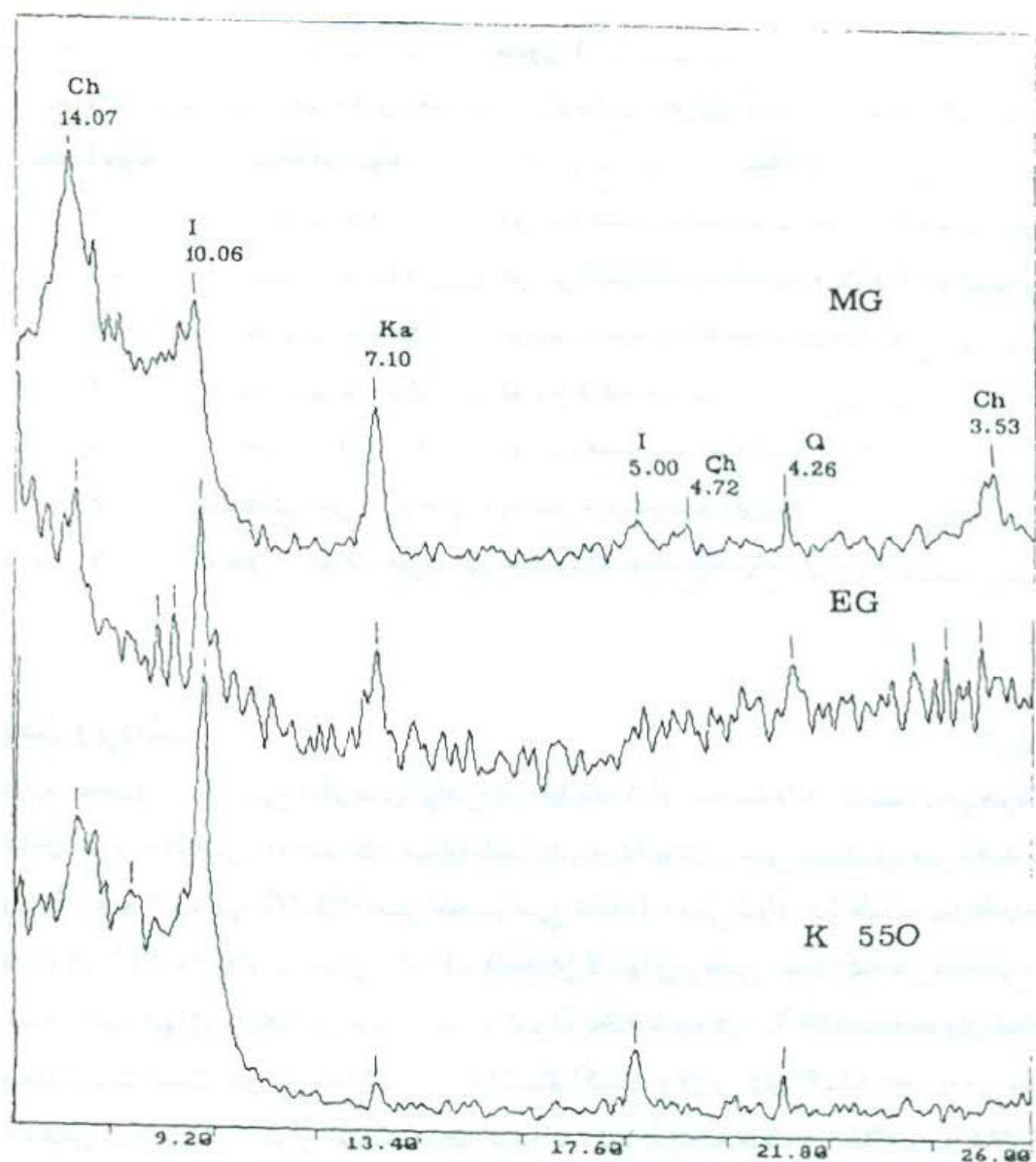
شکل ۱ پراش نگاشت پرتو ایکس ذرات رس. MG منیزیم کلرید، EG تیمار با اتیلن گلیکول، K 550 نمونه حرارت داده شده در کوره. I ایلیت، Ch کلریت، Ka کائولینیت، Q کوارتز
