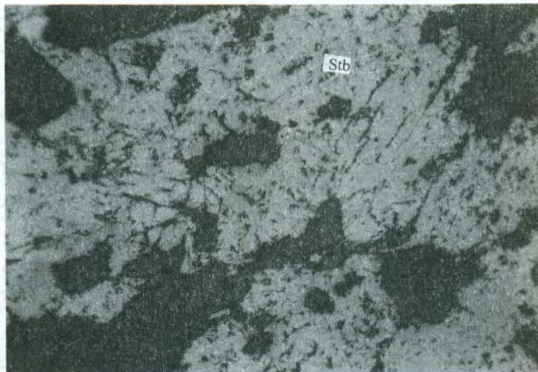
شکل ۳ بلورهای استیینیت (Stb) رگه های فقیره در زیر نور PPL (بزرگنمایی ۱۰۰x).
