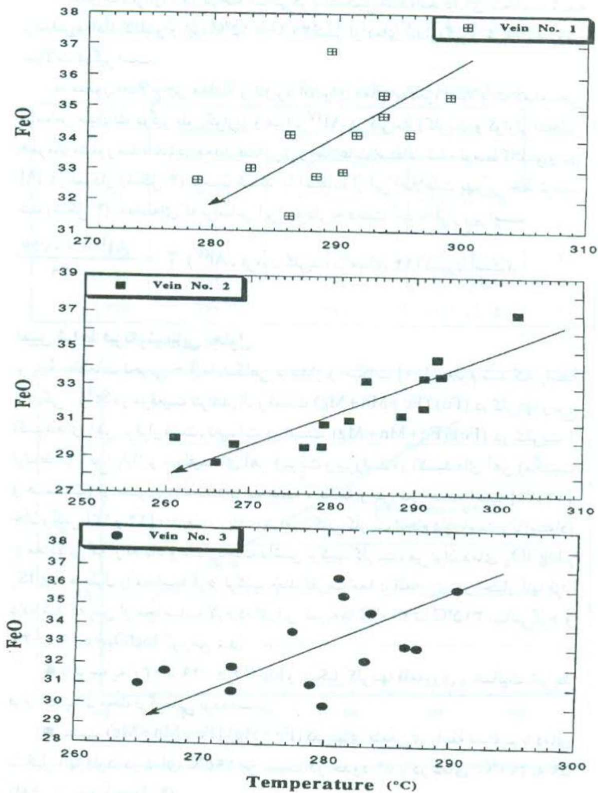
شکل ۵- نمایش بررسی نحوه تغییرات FeO و دما در کلریت‌های قلعه زری
