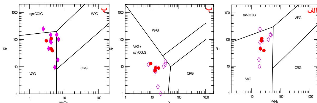
شکل ۱۲ الف، ب و پ) نمودارهای تعیین موقعیت زمین‌ساختی با استفاده از نمودار Nb در مقابل Y، Rb در مقابل Yb+Ta و Rb در مقابل Yb+Ta در مقابل Yb+Ta. [۴۲] بنابر این نمودارها، نمونه‌های مورد بررسی بیشتر در قوس‌های آتشفشانی قرار می‌گیرند (VAG). (ORG = مناطق پشته‌ای اقیانوسی = VAG = مناطق کمان آتشفشانی WPG = مناطق داخل صفحه‌ای COLG = محیط‌های تصادمی) (نمادهای لوزی سنگ‌های درونی و نمادهای دایره سنگ‌های بیرونی).
