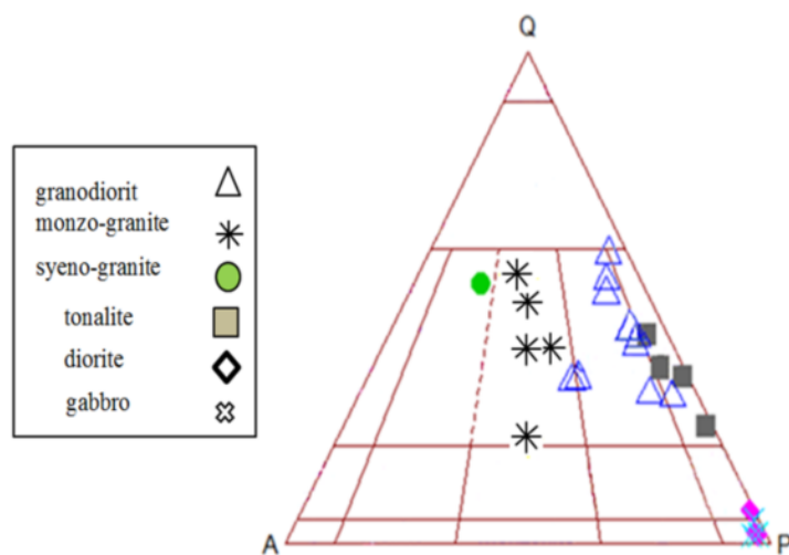
شکل ۳ نمودار رده‌بندی سنگ‌های گرانیوتوئیدی براساس مودال [۱۲]. بنابر این نمودار، نمونه‌ها دارای طیف ترکیبی از سینوگرانیت، مونزوگرانیت، گرانودیوریت، دیوریت و گابرو هستند.
