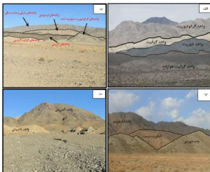
شکل ۲ الف) واحدهای سازنده‌ی گرانیوتوئید چهارفرسخ، در بالاترین بخش، بیشتر گرانودیوریتی و در بخش‌های پایینی دیوریتی هستند. ب) مجموعه‌های فلیشی، سنگ میزبان واحدهای گرانیوتوئیدی، پ) واحدهای گرانیوتوئیدی، واحدهای دگرگونه (آندالوزیت شیست) و واحدهای دیوریتی، منطقه سمافات، ت) واحدهای خروجی آندزیتی و داسیتی واقع در شمال روستای بیچند (نیل چاه و چاه شاهی).
