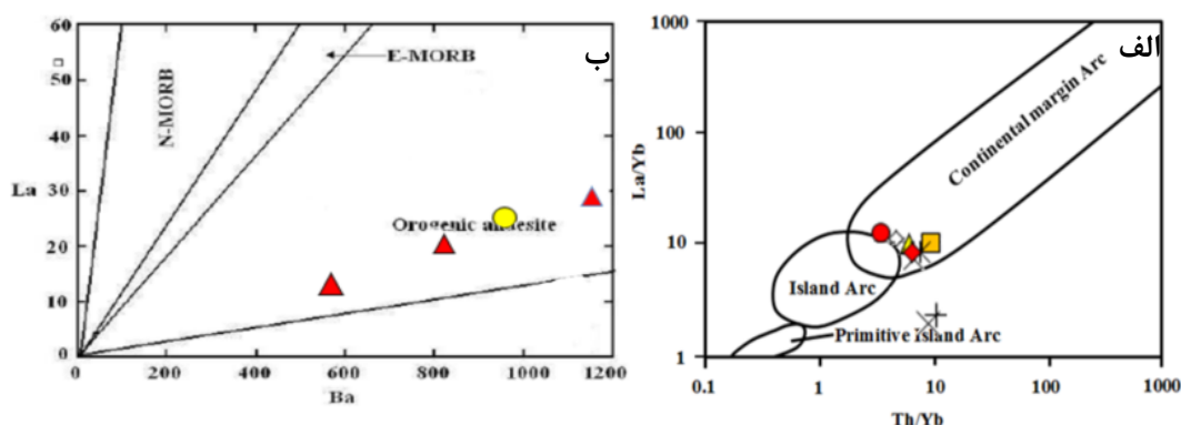
شکل ۱۳ الف) نمودار La/Yb در مقابل Th/Yb [۴۳] برای تعیین محیط زمین‌ساختی توده‌های گرانیتوئیدی مورد بررسی (نشانها مشابه با شکل ۶-ب). الف) ب) تعیین محیط زمین‌ساختی سنگ‌های بیرونی منطقه مورد بررسی [۴۴] بنابر این نمودار، سنگ‌های منطقه‌ای مورد بررسی در گستره‌ی آندزیت‌های ناشی از کوهزایی قرار می‌گیرند (نمادها مشابه با شکل ۶-ب).
