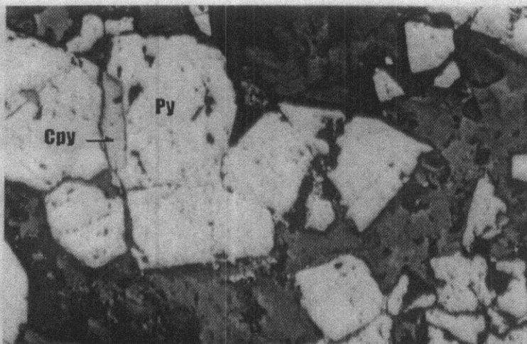
شکل ۴- پر شدن فضای بین بلورهای پیریت تشکیل دهنده بافت پیوندگاه سه گانه با کالکوپیریت (نور عادی) بزرگنمایی \times 100 .
