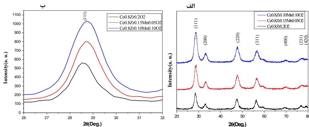
شکل ۱ الف) طرح پراش پرتو X نمونه های سنتز شده در دمای تکلیس 600^{\circ}\text{C} (ب) تصویر بزرگ شده یکی از قله های اصلی در بازه ی زاویه ای 2\theta = 26 - 32^{\circ} .
