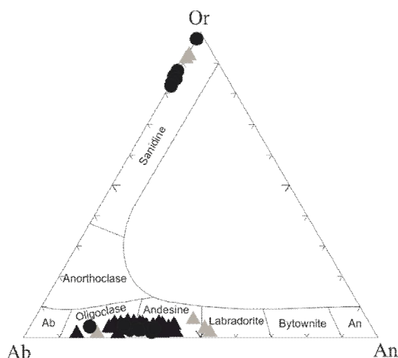
شکل ۱۰ ترکیب فلدسپارهای توده لخشک و دایک‌های درون آن در نمودار (آلبیت) Ab- (آنورتیت) An- (رتوز) Or [۲۲]. گستره ترکیبی فلدسپارها در این سنگ‌ها، بین الیگوکلاز تا آندزین و ارتوز تغییر می‌کند. نمادها مشابه شکل ۶ می‌باشند.
