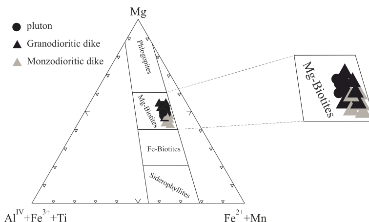
شکل ۶ نمودار رده‌بندی میکاها برپایه‌ی ترکیب شیمیایی آنها [۱۴]. براین اساس تمامی بیوتیت‌های مورد بررسی \text{Mg-Biotite} هستند.
