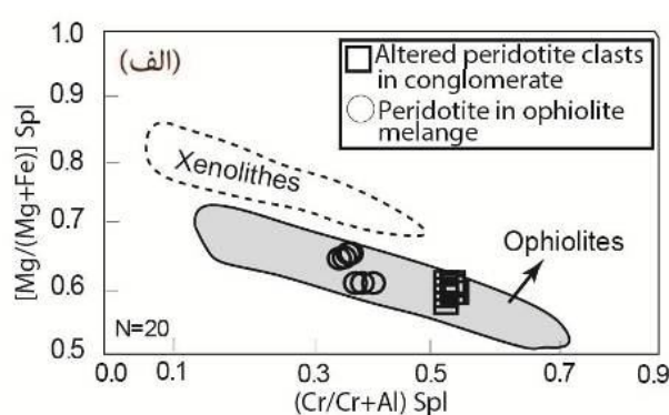
شکل ۴ (الف) نمودار Mg/(Mg+Fe) نسبت به Cr/(Cr+Al) در اسپینل [۱۷، ۱۶]، (ب) نمودار درصد وزنی Al_2O_3 نسبت به Cr_2O_3 اسپینل [۱۸]. ترکیب اسپینل در پریدوتیت‌های مجموعه‌ی افیولیتی پیرانشهر برای مقایسه در نمودار تصویر شده است. ترکیب اسپینل در قطعات پریدوتیت دگرسان شده درون کنگلومرا و پریدوتیت‌های ملانژ افیولیتی پیرانشهر در گستره‌ی آرایه‌ی گوشته‌ای قرار می‌گیرند.
