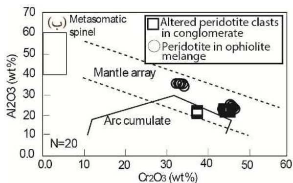
شکل ۴ (الف) نمودار Mg/(Mg+Fe) نسبت به Cr/(Cr+Al) در اسپینل [۱۷، ۱۶]، (ب) نمودار درصد وزنی Al_2O_3 نسبت به Cr_2O_3 اسپینل [۱۸]. ترکیب اسپینل در پریدوتیت‌های مجموعه‌ی افیولیتی پیرانشهر برای مقایسه در نمودار تصویر شده است. ترکیب اسپینل در قطعات پریدوتیت دگرسان شده درون کنگلومرا و پریدوتیت‌های ملانژ افیولیتی پیرانشهر در گستره‌ی آرایه‌ی گوشته‌ای قرار می‌گیرند.
