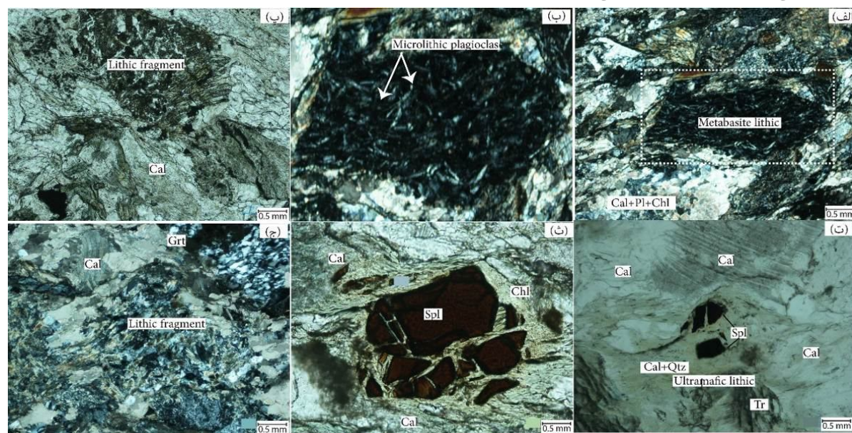
شکل ۳ (الف) کنگلومرا با بافت برشی. قطعه‌ی بازالت با میکرولیت‌هایی از پلاژیوکلاز از دو طرف کشیدگی نشان می‌دهد. کلسیت به همراه کوارتز و کلریت ریزدانه در زمینه‌ی برشی قابل تشخیص است، حالت XPL، (ب) میکرولیت‌های پلاژیوکلاز در قطعات بازالتی، حالت XPL، (پ) کلسیت تشکیل دهنده اصلی زمینه‌ی کنگلومرا، حالت PPL، (ت) بقایای اسپینل در قطعات پریدوتیت دگرسان شده با زمینه‌ی کلسیتی و کمتر کوارتز، حالت PPL، (ث) بقایای اسپینل به رنگ سرخ قهوه‌ای. زمینه سنگ از کلسیت تشکیل شده است، حالت PPL، (ج) کانی‌های ثانویه کوارتز و گارنت در قطعات پریدوتیت دگرسان شده. بافت برشی در زمینه‌ی سنگ مشخص است، حالت XPL.
