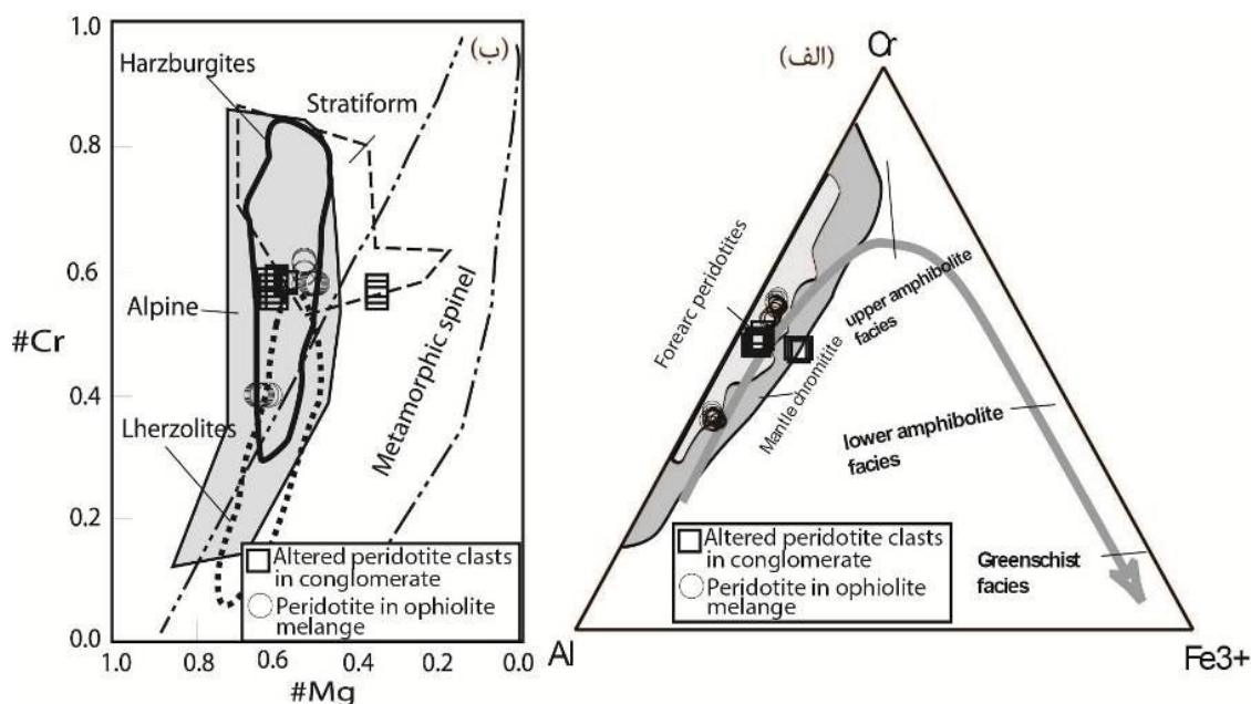
شکل ۵ (الف) ترکیب اسپینل در نمودار مثلثی \text{Cr-Al-Fe}^{3+} [۱۹]، (ب) نمودار \#Cr در مقابل \#Mg (گستره‌های هارزبورژیت و لرزولیت از [۲۰] و گستره‌های آلپی و لایه‌ای از شکل [۲۱]). ترکیب اسپینل در قطعات پریدوتیت دگرسان درون کنگلومرا قابل مقایسه با پریدوتیت‌های ملانژ افیولیتی پیرانشهر در گستره‌ی آلپی قرار می‌گیرند. بر اساس \#Cr اسپینل ترکیب سنگ مادر در قطعات پریدوتیت دگرسان کنگلومراهای مورد بررسی از نوع هارزبورژیتی تعیین می‌شود.
