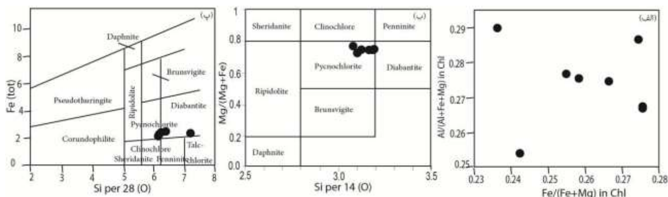
شکل ۷ ترکیب کلریت در قطعات پریدوتیتی دگرسان شده در کنگلومراهای پیرانشهر. (الف) نمودار Al/(Al+Fe+Mg) در مقابل Fe/(Fe+Mg) . (ب) نمودار کاتیونی Si در مقابل Mg/(Mg+Fe) [۲۲]، (پ) نمودار Si در مقابل Fe\ (tot) [۲۲]. کلریت‌های تجزیه شده دارای مقادیر بالای Mg بوده و در نمودارهای رده‌بندی ترکیب آنها در گستره‌ی پیکنولکر و دیابانتیت قرار می‌گیرند.
