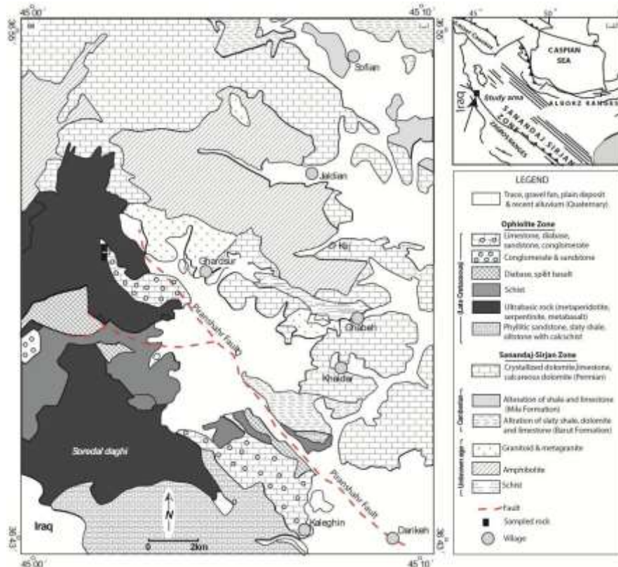
شکل ۱ (الف) موقعیت منطقه‌ی مورد بررسی در تقسیم‌بندی‌های ساختمانی ایران، (ب) نقشه‌ی زمین‌شناسی منطقه‌ی مورد بررسی (با اقتباس از نقشه زمین‌شناسی ۱/۱۰۰۰۰۰ [۱۴]).
