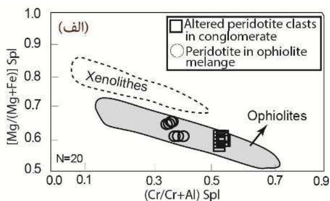
شکل ۴ الف) نمودار Mg/(Mg+Fe) نسبت به Cr/(Cr+Al) در اسپینل [۱۷، ۱۶]، ب) نمودار درصد وزنی Al_2O_3 نسبت به Cr_2O_3 اسپینل [۱۸]. ترکیب اسپینل در پریدوتیت‌های مجموعه‌ی افیولیتی پیرانشهر برای مقایسه در نمودار تصویر شده است. ترکیب اسپینل در قطعات پریدوتیت دگرسان شده درون کنگلومرا و پریدوتیت‌های ملانژ افیولیتی پیرانشهر در گستره‌ی آرایه‌ی گوشته‌ای قرار می‌گیرند.
