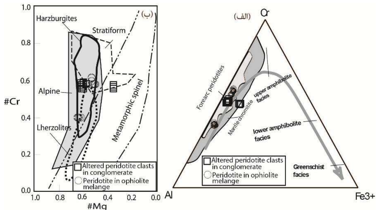
شکل ۵ (الف) ترکیب اسپینل در نمودار مثلثی Cr-Al-Fe^{3+} [۱۹]، (ب) نمودار \#Cr در مقابل \#Mg (گستره‌های هارزبوریت و لرزولیت از [۲۰] و گستره‌های آلپی و لایه‌ای شکل از [۲۱]). ترکیب اسپینل در قطعات پریدوتیت دگرسان درون کنگلومرا قابل مقایسه با پریدوتیت‌های ملانژ افیولیتی پیرانشهر در گستره‌ی آلپی قرار می‌گیرند. بر اساس \#Cr اسپینل ترکیب سنگ مادر در قطعات پریدوتیت دگرسان کنگلومراهای مورد بررسی از نوع هارزبوریتی تعیین می‌شود.
