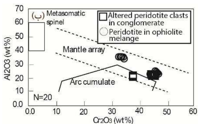
شکل ۴ الف) نمودار Mg/(Mg+Fe) نسبت به Cr/(Cr+Al) در اسپینل [۱۷، ۱۶]، ب) نمودار درصد وزنی Al_2O_3 نسبت به Cr_2O_3 اسپینل [۱۸]. ترکیب اسپینل در پریدوتیت‌های مجموعه‌ی افیولیتی پیرانشهر برای مقایسه در نمودار تصویر شده است. ترکیب اسپینل در قطعات پریدوتیت دگرسان شده درون کنگلومرا و پریدوتیت‌های ملانژ افیولیتی پیرانشهر در گستره‌ی آرایه‌ی گوشته‌ای قرار می‌گیرند.
