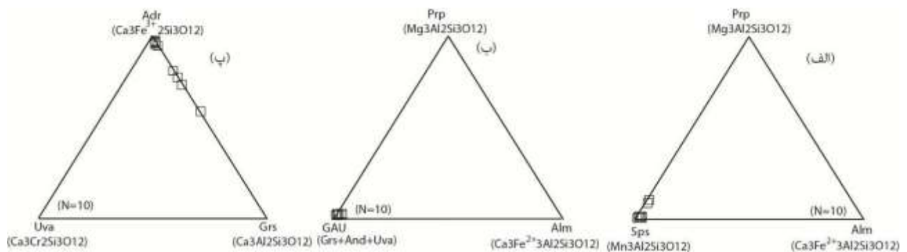
شکل ۶ ترکیب گارنت در قطعات پدیدوتیتی دگرسان شده کنگلومراهای مجموعه‌ی دگرگونی پیرانشهر. (الف) نمودار Sps-Prp-Alm ترکیب فقیر از \text{Fe}^{2+} و Mg گارنت را نشان می‌دهد، (ب) در نمودار Prp-Alm-(Grs+And+Uva) ترکیب گارنت در راس GAU، (ج) در نمودار Grs-Adr-Uva ترکیب گارنت روی ضلع Adr-Grs قرار می‌گیرند. بر این اساس ترکیب گارنت‌های مورد بررسی فقیر از کروم هستند.
