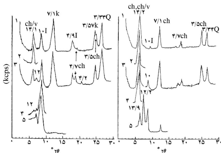
شکل ۱ پراش نگاشت پرتو ایکس ذرات رس افق A1 (۱۳-۰ نیمرخ خاک ۱). شکل ۲ پراش نگاشت پرتو ایکس ذرات رس افق C (۱۷۵-۱۲۲، نیمرخ خاک ۱). (آنالیز بعضی تیمارها (۲ و ۴ و ۵ در شکل ۱ و ۲) در زاویه محدود به 2\theta صورت گرفته است). پراش نگاشت ۱: نمونه اشباع شده با منیزیم پراش نگاشت ۲: نمونه ۱ + گلیکول پراش نگاشت ۳: نمونه اشباع شده با پتاسیم پراش نگاشت ۴: نمونه ۳ + دمای 350^{\circ}\text{C} به مدت ۲ ساعت پراش نگاشت ۵: نمونه ۳ + دمای 550^{\circ}\text{C} به مدت ۲ ساعت (اعداد روی قله ها به انگستروم) S = اسمکتیت I = ایلیت ch = کلریت Q = کوآرتز K = کائولینیت V = ورمیکولیت mi = میکا
