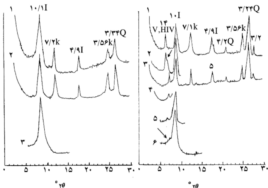
شکل ۵ پراش نگاشت پرتو ایکس ذرات رس افق ۱ Bxg (۱۰۷-۶۷ نیمرخ خاک ۲).
