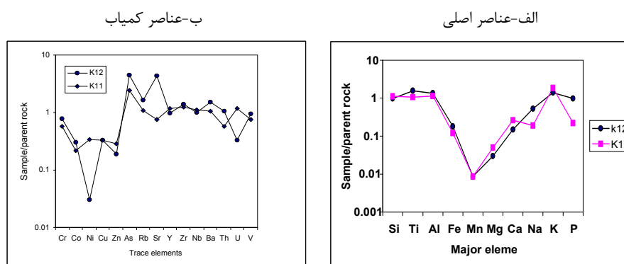
شکل ۸ الگوهای عناصر (الف) اصلی و (ب) عناصر کمیاب در کانسار خاک نسوز کبوترکوه گناباد، نرمال شده با سنگ مادر (آندزیت‌های منطقه).
