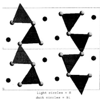
شکل ۶ ساختار چهاروجهی هرم‌های سه‌گوش به موازات (010) در \text{CuSbS}_4 که با EXAFS از کانی چلکستیپایت سنتز شده در 450^\circ\text{C} به دست آمده است.
