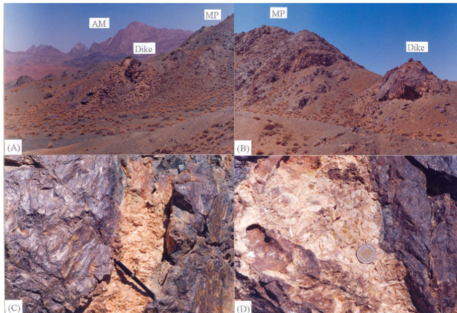
شکل ۳ تصاویر صحرایی رودینگیت‌های موجود در افیولیت شمال انارک (شمال شرق استان اصفهان). (A): دایک رودینگیتی شده درون پریدوتیت‌های سرپانتینی شده گوشته (MP)، و دگرگونه‌های انارک (AM) (نگاه به شمال). (B): دایک رودینگیتی درون پریدوتیت‌های سرپانتینی شده گوشته، در جنوب شرقی چاه درختک (نگاه به جنوب). (C) و (D): رودینگیت‌های رگه‌ای (بخش روشن) در درون رودینگیت‌های توده‌ای (بخش تیره).
