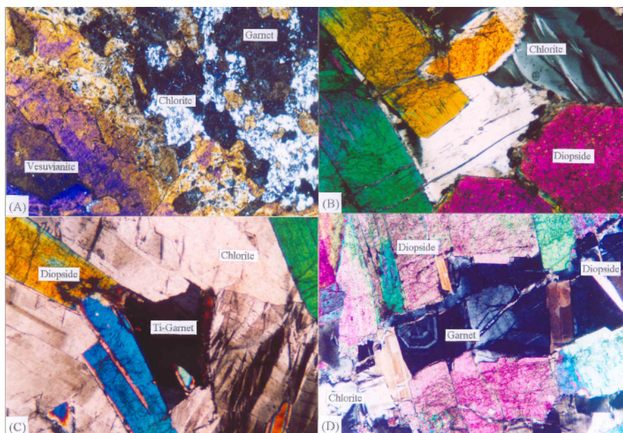
شکل ۴ تصاویر میکروسکوپی رودینگیت‌های افیولیت شمال انارک (شمال شرق استان اصفهان) (بزرگنمایی ۲۰ برابر). (A): تصویری از رودینگیت‌های توده‌ای با کانی‌های گارنت، وزوینیت (ایدوکراز)، و کلریت. (B) و (C): تصویر رودینگیت‌های رگه‌ای فاز اول با کانی‌های دیوپسید، کلریت، و گارنت تیتان‌دار. (D): رودینگیت رگه‌ای فاز دوم با کانی‌های گارنت، کلریت و دیوپسید، که رودینگیت رگه‌ای فاز اول را قطع کرده است.
