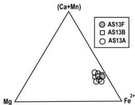
شکل ۳ ترکیب شیمیایی گارنت های مطالعه شده در نمودار سه تایی Mg ، Fe^{2+} ، Mn+Ca . آلماندن مهمترین عضو نهایی است و مقداری گروسولار و اسپسارتین نیز وجود دارد.
