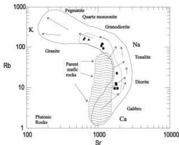
شکل ۷ نمودار لگاریتمی Rb بر حسب [^{87}Sr] . سنگهای آذرین درونی که با تفریق گرمابی تشکیل شده‌اند، غنی‌شدگی نسبی از K ، Na و Ca را نشان می‌دهند. پیکانها روند تفریق گرمابی را نشان می‌دهند و نمونه‌های پنج کوه نیز جهت مقایسه با علائم شبیه شکل ۶ آورده شده‌اند.
