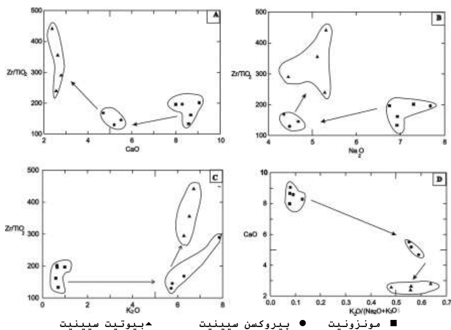
شکل ۶ نمودارهای Zr/TiO_2 برحسب (A) CaO ، (B) Na_2O و (C) K_2O ، و نیز CaO بر حسب (D) K_2O / (Na_2O + K_2O) برای نمونه‌های پنج کوه. به جهت پیکانها که نشان‌دهنده مسیر دگرسانی مونزونیت به پیروکسن سینیت و بیوتیت سینیت‌اند توجه شود.
