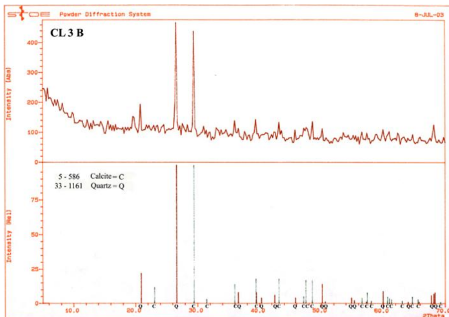
شکل ۶ طرح XRD نمونه CL3B پس از پخت‌درمانی.
