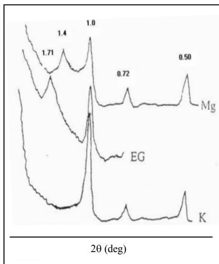
شکل ۸. انتقال موفقیت آمیز هیدروکسیدهای بین لایه ای بوسیله تیمار سوم (اسید کلریدریک، دمای °C ۴۰۰ و سود نیم نرمال در حال جوش) و انبساط پیک ۱/۴ نانومتر به ۱/۷۱ نانومتر پس از تیمار اتیلن گلیکول.
