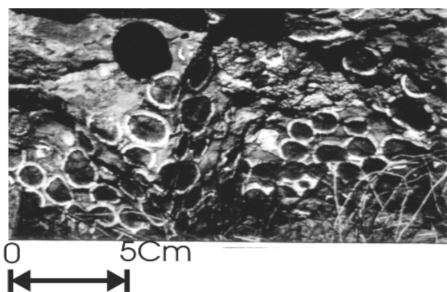
شکل ۳ لیستونیت سیلیسی (Lv) به صورت یک ورقه بر روی سرپانتینیت (Serp) (جنوب کلاته سلیمان).
