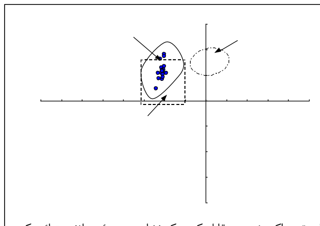
شکل ۷ تغییرات ایزوتوپ اکسیژن در مقابل کربن که نشان دهنده دیانتر متاوریکی در سازند ایلام است. در این نمودار محدوده سنگ آهک‌های دریایی کرتاسه [۹] و محدوده آهک‌های آب‌های کم عمق هولوسن [۱۳] مشخص شده است.
