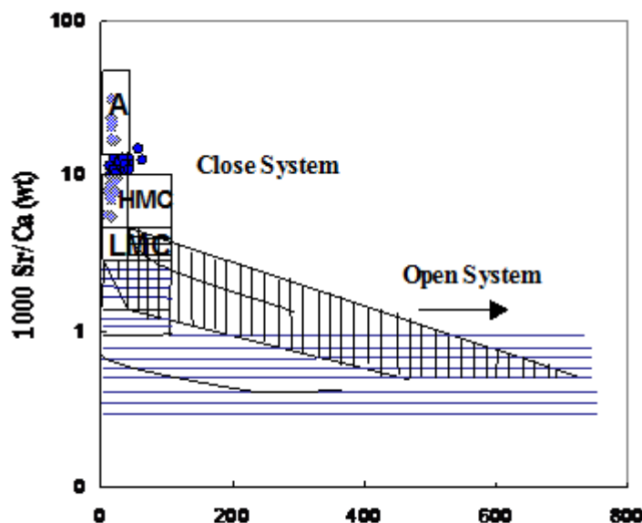
شکل ۶ نسبت مقادیر Sr/Ca در مقابل Mn محدوده‌های تعیین شده توسط برند و وایزر [۵] اغلب نمونه‌های آهکی سازند ایلام تحت تاثیر فرایندهای دیاژنتیکی در یک سیستم بسته تا نیمه بسته قرار گرفته‌اند.
