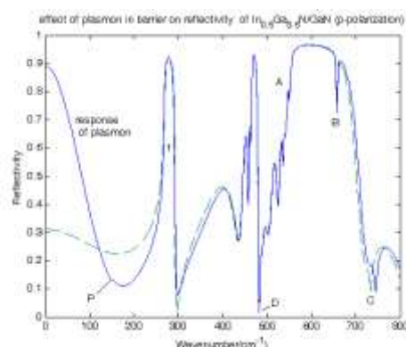
شکل ۸ طیف بازتابی چاه کوانتومی \text{In}_{0.5}\text{Ga}_{0.5}\text{N}/\text{GaN} ناآلاییده با قطبش P و زاویه تابش 12^\circ .
