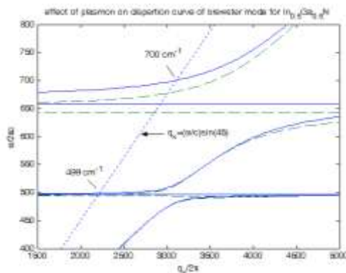
شکل ۳ منحنی پاشیدگی مد بروستر آلیاژ \text{In}_{0.5}\text{Ga}_{0.5}\text{N} آلانئید (منحنی توپر) و ناآلانئید (منحنی خط چین).
