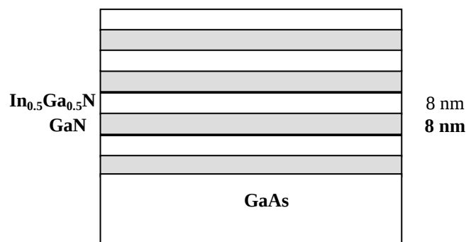
شکل ۷ نمایی از MQW روی زیر لایه GaAs.
