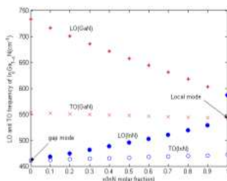
شکل ۵ بسامدهای طولی و عرضی آلیاژ \text{In}_x\text{Ga}_{1-x}\text{N} به ازای مقادیر مختلف x.
