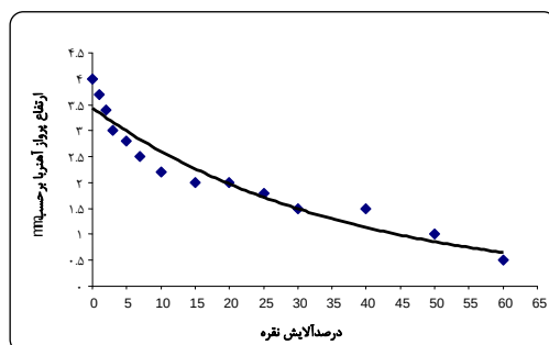
شکل ۱ تغییرات ارتفاع آهن‌ربا از سطح نمونه بر حسب درصد آلاینش در نمونه‌های سری اول در دمای در حدود 77\text{ K} .
