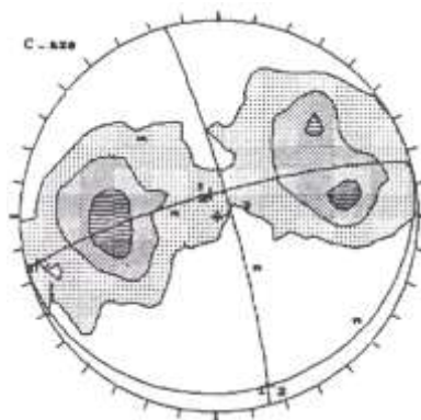
شکل ۷ نمودار پربندی محور نوری دانه‌های کوارتز (N260/55 و N75/40).
