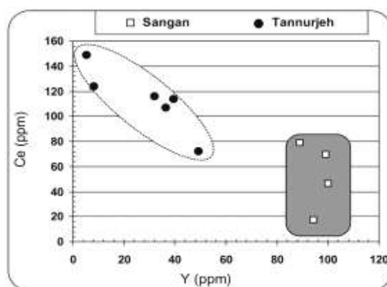
شکل ۱۱ مقایسه Ce-Y نمونه‌های سنگ منشأ سنگان و تنورجه.
