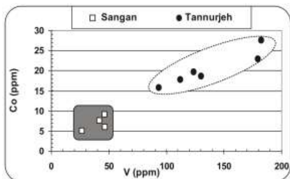
شکل ۷ مقایسه Co-V نمونه‌های سنگ منشأ سنگان و تنورجه.
