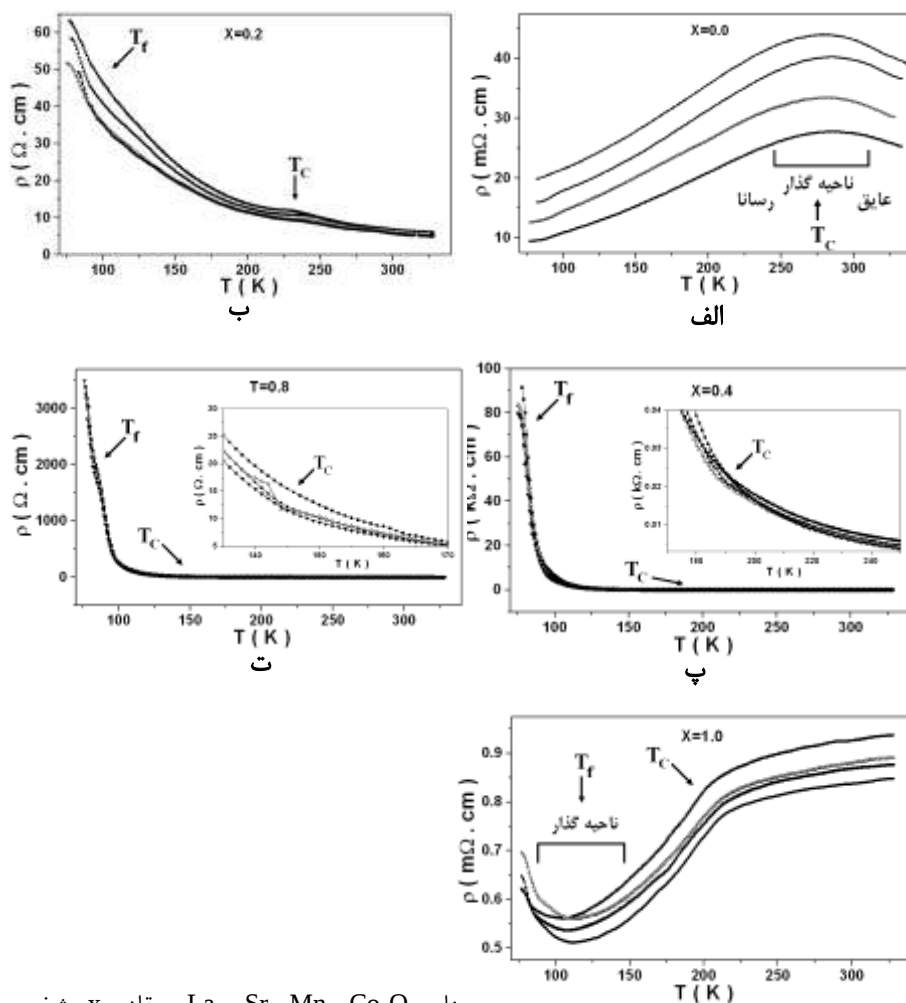
شکل ۳. بستنی همبستگی و پیرامونی همبستگی برای \text{La}_{0.7}\text{V}_{0.3}\text{Sr}_{1-x}\text{Mn}_{1-x}\text{Co}_x\text{O}_3 و مقادیر x مشخص شده روی هر شکل که در حضور میدانهای مغناطیسی خارجی ثابت اندازه‌گیری شده‌اند ( \blacksquare : H = 0 \text{ Oe} , \bullet : H = 5 \text{ kOe} , \Delta : H = 10 \text{ kOe} , \blacktriangledown : H = 15 \text{ kOe} ). T_C دمای گذار فرومغناطیس به پارامغناطیس و T_f دمای گذار حالت اسپین کم به حالت اسپین متوسط کبالت را نشان می‌دهد.
