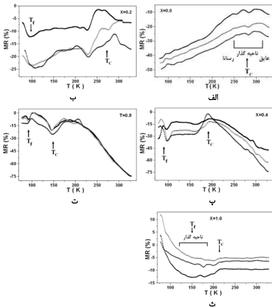
شکل ۷ بستگی دمایی مغناطومتقاومت نمونه‌های \text{La}_{0.70}\text{Sr}_{0.30}\text{Mn}_{1-x}\text{Co}_x\text{O}_3 در حضور میدانهای مغناطیسی خارجی مختلف ( \blacksquare : H = 0 Oe, \circ : H = 5 kOe, * : H = 10 kOe).
