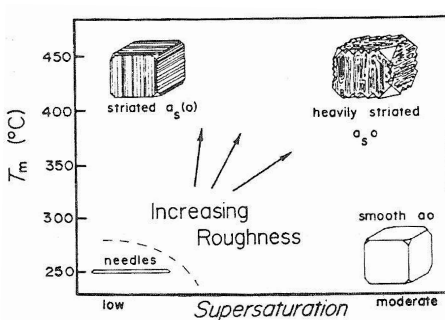
شکل ۳ اشکال مختلف رشد بلوری در کانی پیریت و در شرایط گرمایی T_m = دمای متوسط، a = (100) ، o = (111) ، شیار دار s = [6] . o = (111) سطوح با گسترش کمتر.
