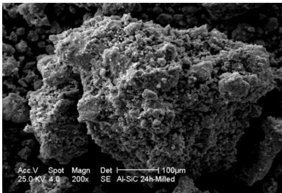
شکل ۳- تصویر میکروسکوپ الکترونی روبشی یک ذره آلومینیم کلوخته‌ای شده پس از ۲۴ ساعت آسیاب‌کاری.
