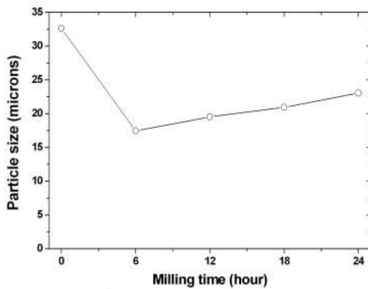
شکل ۶ تغییر اندازه متوسط ذرات ( D_{10} ) با زمان آسیاب‌کاری.
