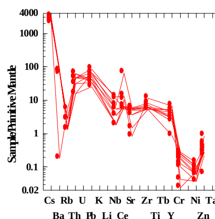
شکل ۱۹ الگوی عناصر جزئی نمونه‌های
