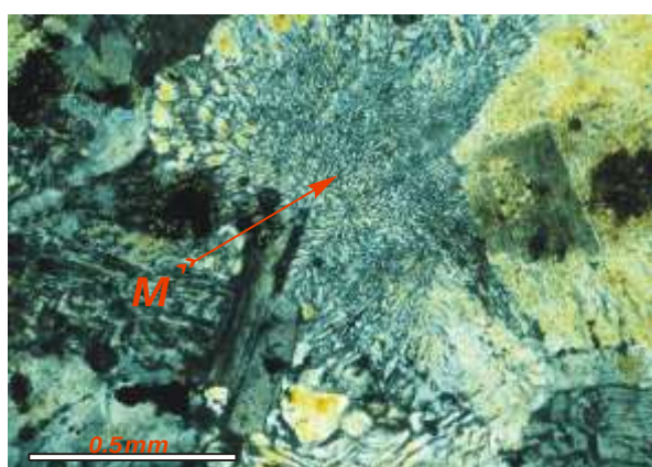
شکل ۱۳ نمونه‌های پلاژیوگرانیتی با بافت گرافیک از نوع گرانوفیری.
