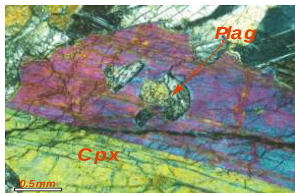
شکل ۱۰ درشت بلورهای کلینوپیروکسن (Cpx) و پلاژیوکلاز (Plag) در گابروهای پگماتوئیدی.
