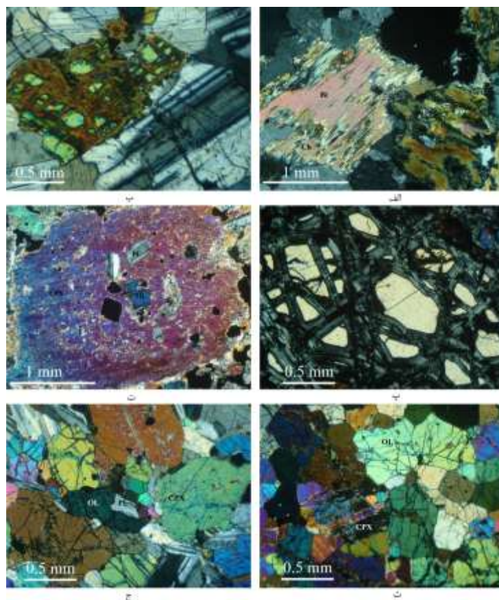
شکل ۳ الف) دگرش بلورهای بیوتیت به بلورهای کلریت و اپیدوت در نمونه پلاژیوگرانیت (XPL, F.W, 1.75*2.5 mm 2 ب) شکستگی بلور پلاژیوکلز در اثر پدیده سرپانتینی شدن بلورهای الیوین در نمونه تروکتولیتی (XPL, F.W, 1.75*2.5 mm 2 پ) بافت باقیمانده در نمونه دونیتی (XPL, F.W, 1.75*2.5 mm 2 ت) بافت پوئی کلریتیک در بلورهای کلینوپیروکسن (XPL, F.W, 1.75*2.5 mm 2 ث) بافت ادکومولا در نمونه دونیت (XPL, F.W, 0.75*1 mm 2 ج) بافت ارتوکومولا در نمونه الیوین گابرو (XPL, F.W, 0.75*1 mm 2 Bi) = بیوتیت، Ch = کلریت، Ep = اپیدوت، Ol = الیوین، Cpx = کلینوپیروکسن، pl = پلاژیوکلز).
