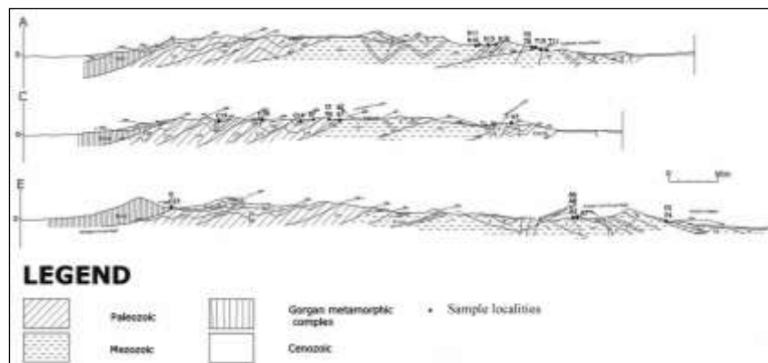
شکل ۳ برش‌های زمین‌شناسی از مسیر دامغان-گرگان [۱۲] که روی آنها موقعیت نمونه‌های به‌کار رفته در تحلیل ریزساختاری و کرنش در این بررسی نشان داده شده است. مسیر برشها در شکل ۱ دیده می‌شود. مقیاس افقی و قائم برشها یکسان است.
