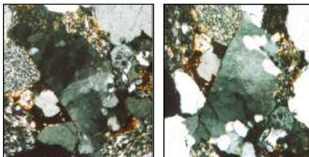
شکل ۶ ریزساختار Sub grain rotation recrystallization که به ترتیب با چرخش میز میکروسکوپ sub grain هایی که در حال تبدیل به یک دانه مجزا هستند به گونه ای واضحتر نمایان می شوند، XPL, 6.3x.
