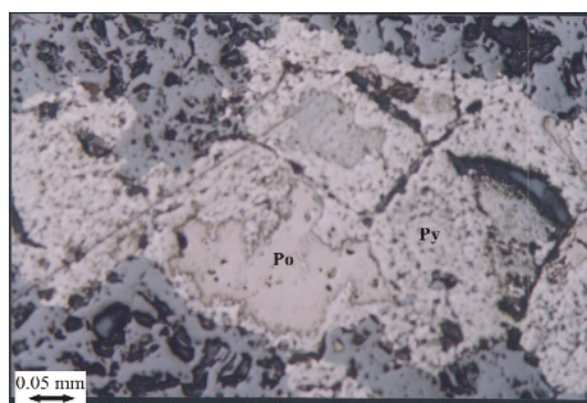
شکل ۱۱ پیریت نسل سوم حاصل از پیروتیت، نور بازتابی و PPL.
