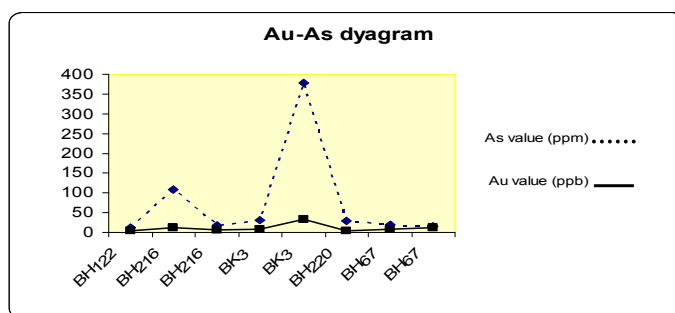
شکل ۳ رابطه مستقیم Au-As در نمونه‌هایی از کانسنگ توده C و باغک.
