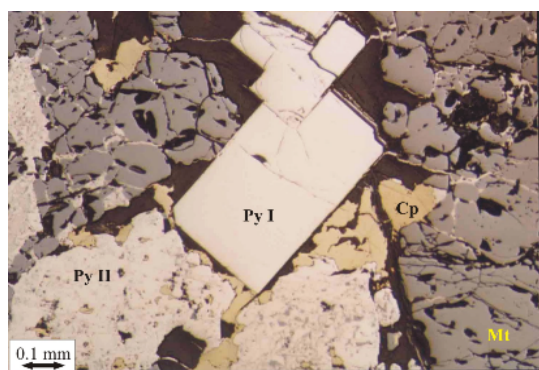
شکل ۱۰ پیروتیت‌های یوهیدرال نسل اول (Py I) و پیروتیت‌های آن هیدرال نسل دوم (Py II)، نور بازتابی و PPL.
